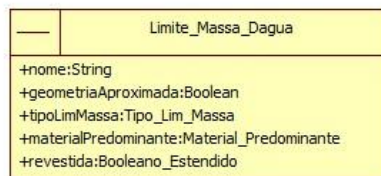
Figura 2-7 – Classe Georreferenciada com Primitiva Geométrica Linha.
