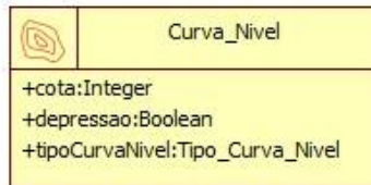
Figura 2-12 – Classe Georreferenciada do tipo Isolinhas.
